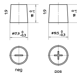
Anschlusspole 1
